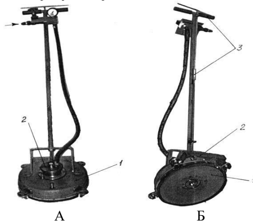
Рисунок 1 – Моющее устройство
