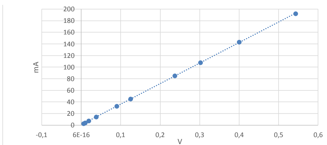
Рис. 2 . Вольт-амперная характеристика образца № 1.
